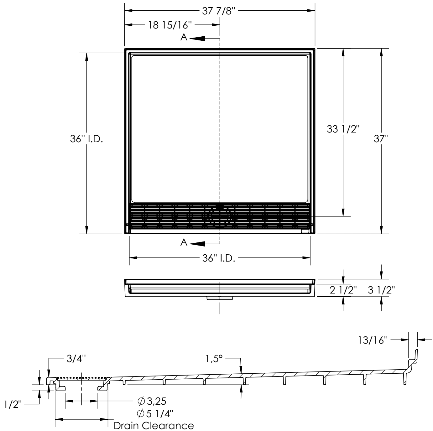
Section A-A
